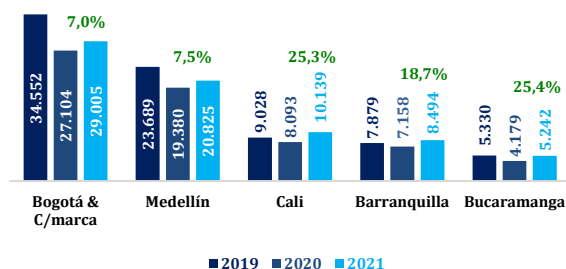
Gráfico 10. Área en proceso* de obra según censo - principales ciudades** (miles m 2 ) 2019-2021
