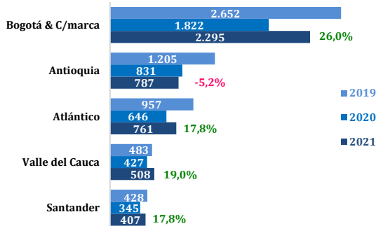
Gráfico 4. Producción de concreto premezclado principales departamentos* (miles de m 3 ) 2019-2021
