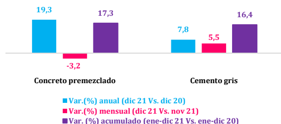
Gráfico 1. Variación anual, mensual y acumulada de la producción de concreto premezclado y cemento gris en Colombia (%) diciembre (2021 Vs. 2020)
